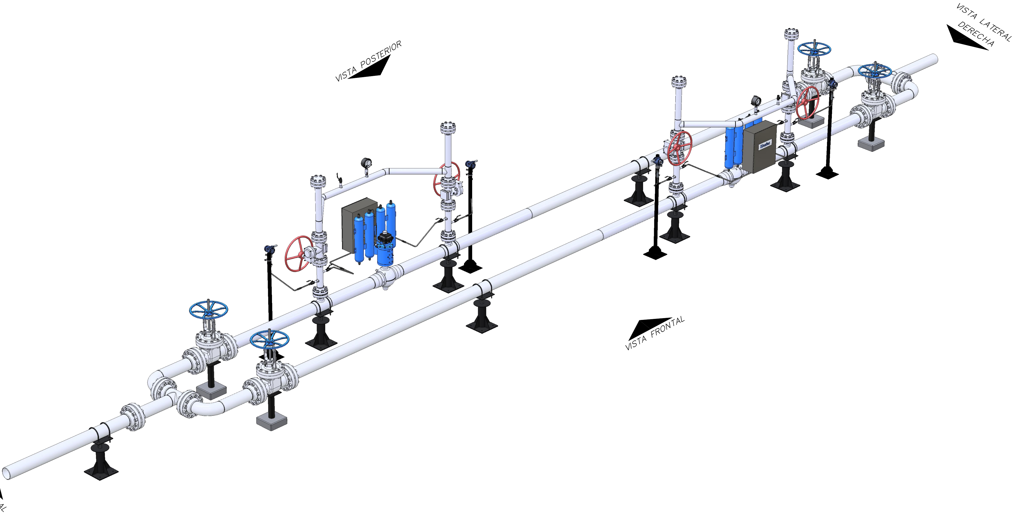
VISTA ISOMÉTRICA ESDV 211-221
